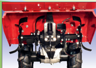
Hacksatz mit geschmiedeten Messern fraise avec couteaux forgés
