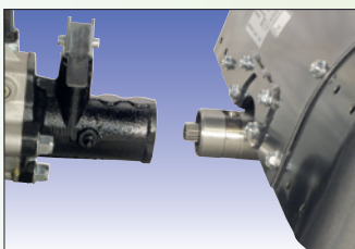
Schnellkupplung für Anbaugeräte
