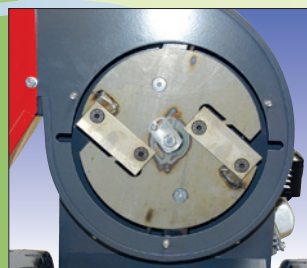
Schnittscheibe mit 2 Messer disque de coupe à 2 couteaux
